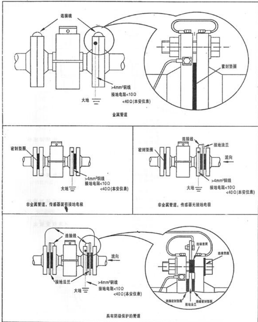
图七 流量计与管道的接地
